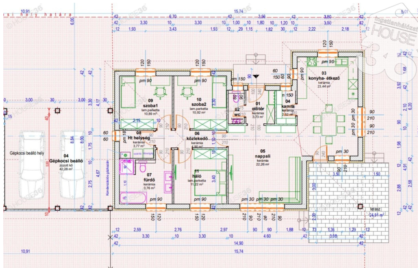
Alaprajz
