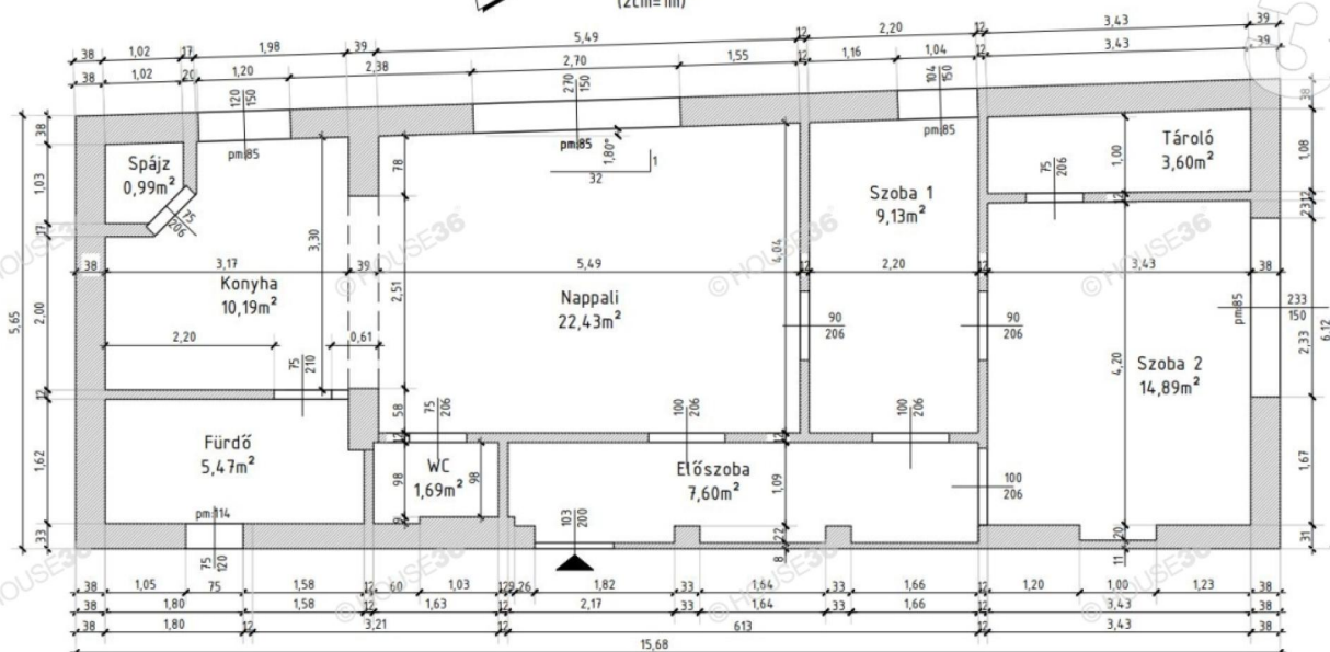
Alaprajz I. em 2: 1:50 (2cm=1m)
