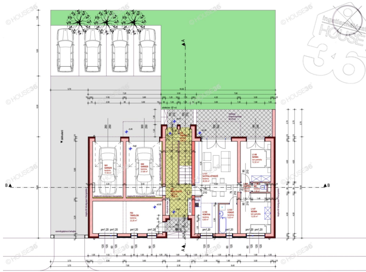
Alaprajz
